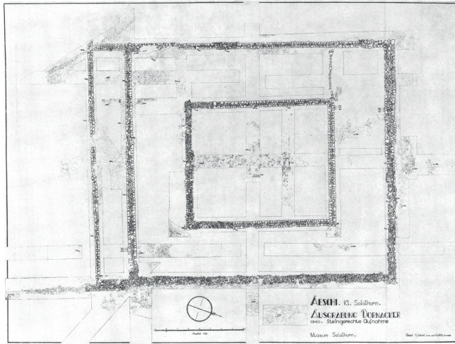
Abb. 2: Steingerechte Aufnahme.
