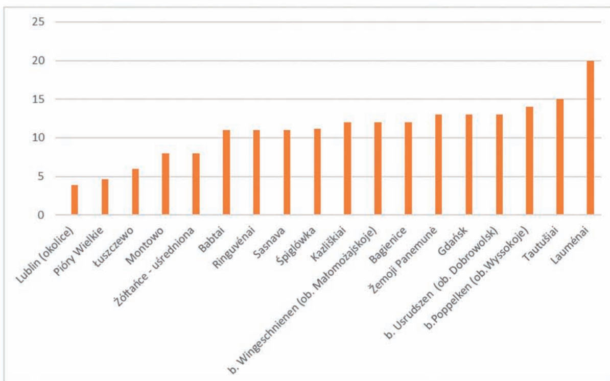
Ryc. 7. Procentowa zawartość a) miedzi (Cu) – w porządku malejącym – i b) cyny (Sn) – w porządku rosnącym – w wybranych siekierkach typu Tautušiai, odmiany C – literatura patrz tabela 1 (oprac. J. Urban)
